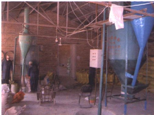
饲料厂饲料加工车间
