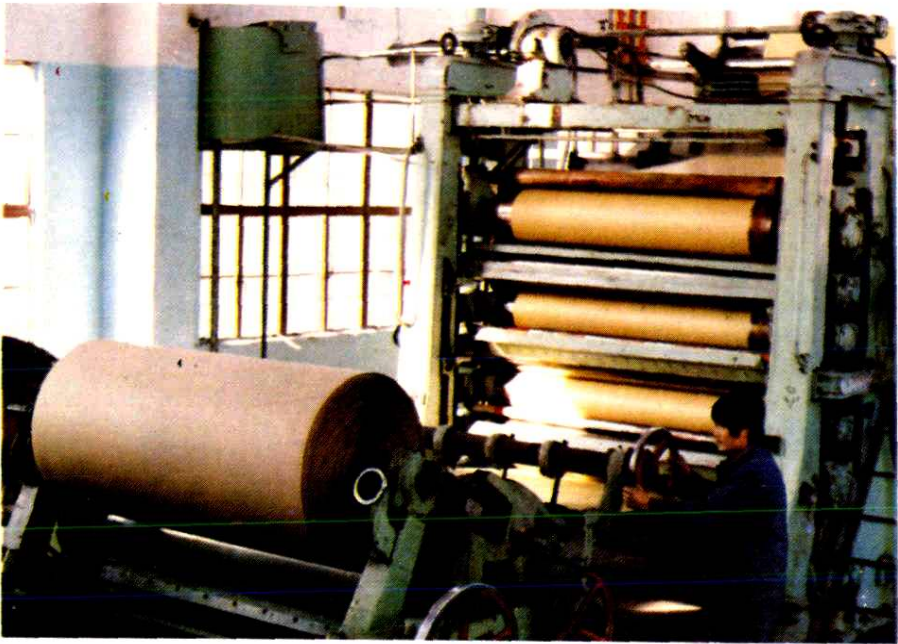
泾县建华造纸厂四号造纸机
