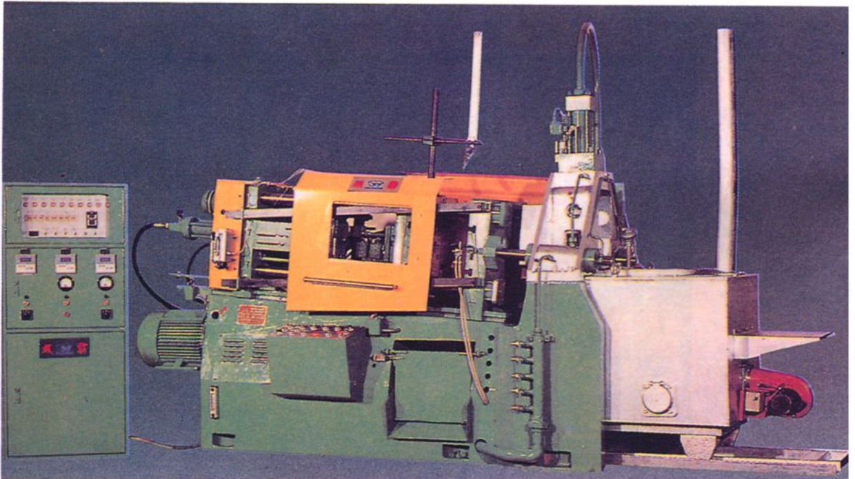
高明县第一机械厂产品——全自动热室锌合金压铸机
