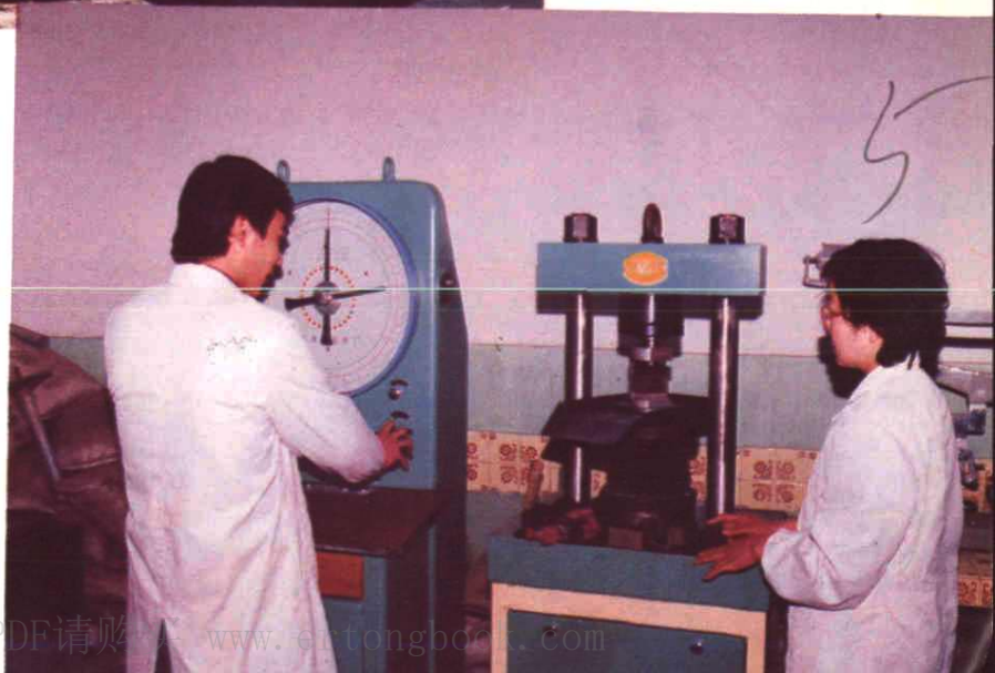
水泥抗压强度测试
