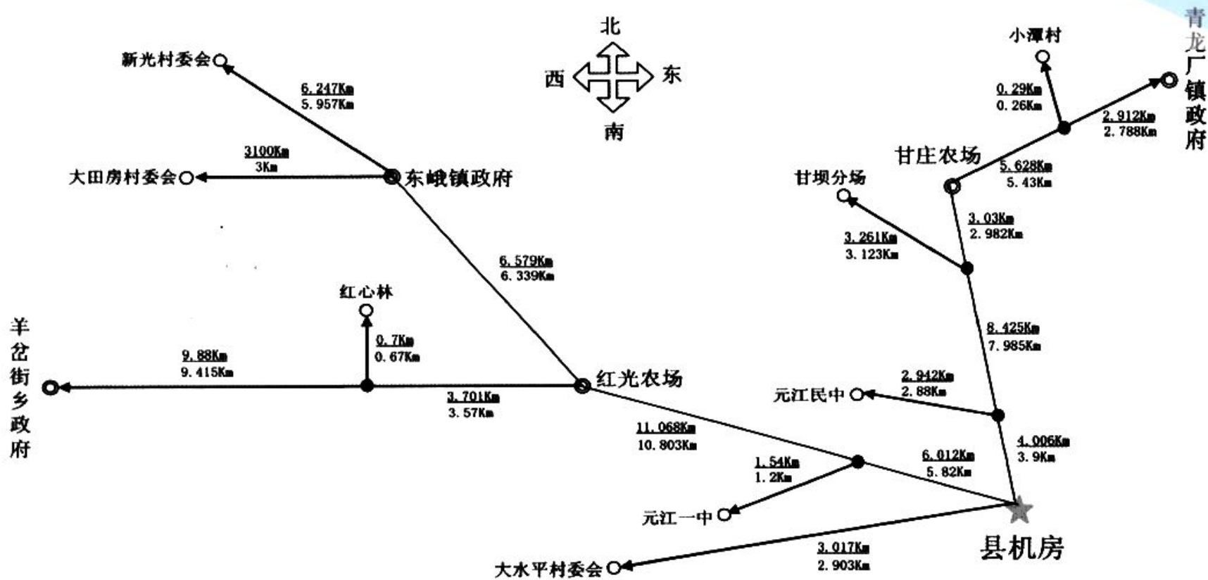
乡镇有线电视光缆路由图2
