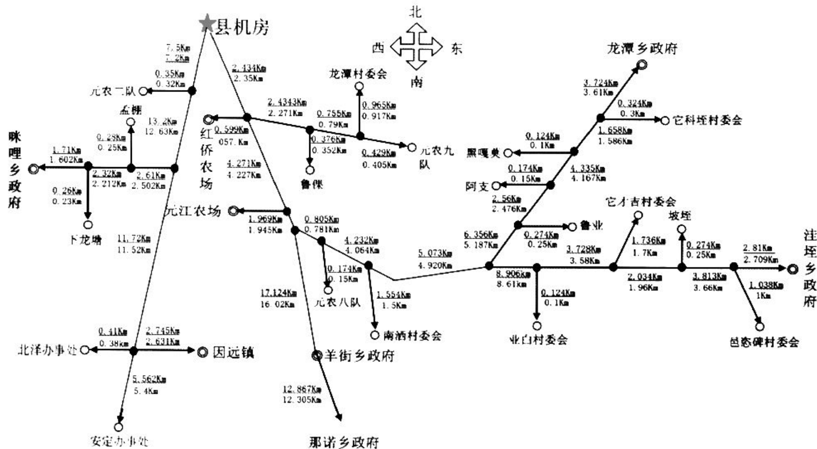
乡镇有线电视光缆路由图 1
