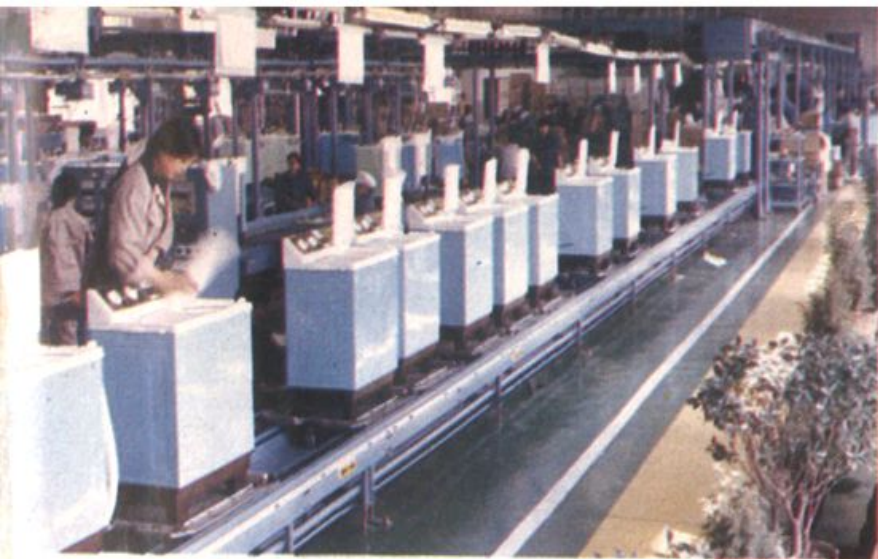
君子兰牌双桶洗衣机 总装车间生产线
