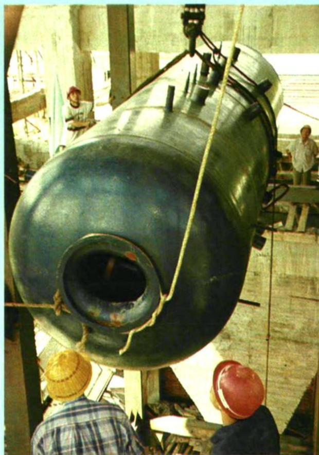
锅炉汽包吊装
