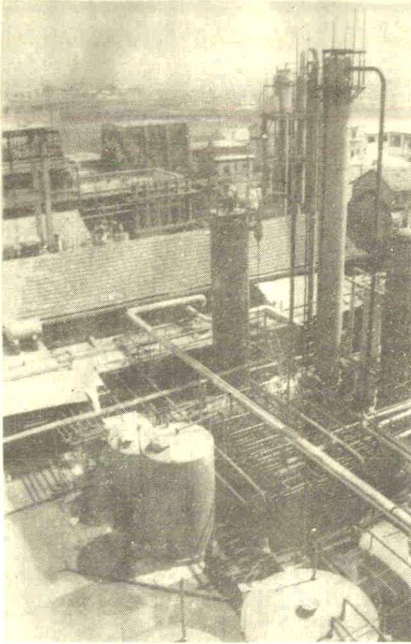
义乌化工厂·碳氨车间一角（吴玉玲摄）
