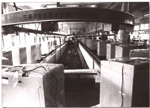
南京电子管厂三乐牌全自动洗衣机自动生产线 (1991 年摄)
