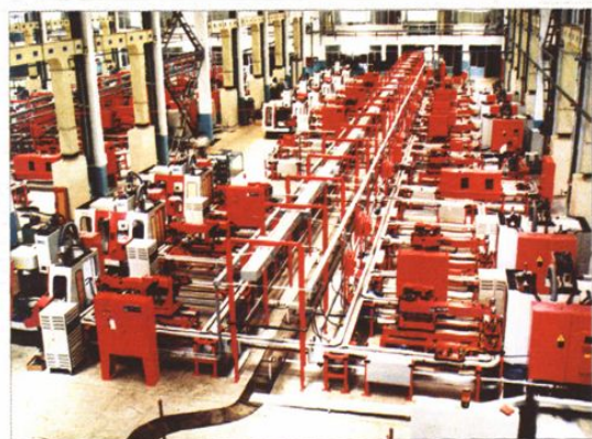
金城集团 1996 年从国外引进的国内第一条摩托车智能化柔性装配线
