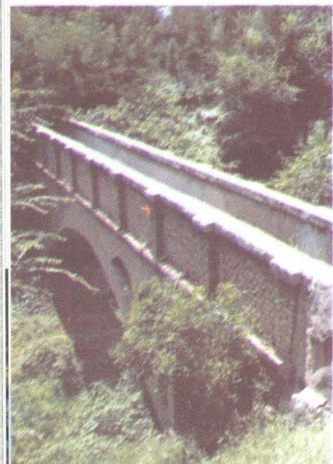
胜利渠渡槽
