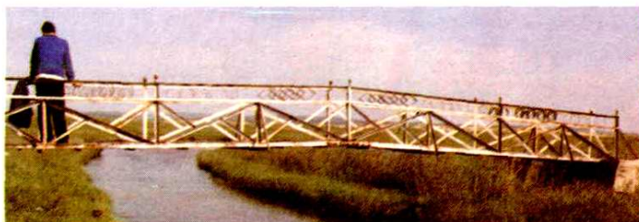
白城子站钢架桥▽
