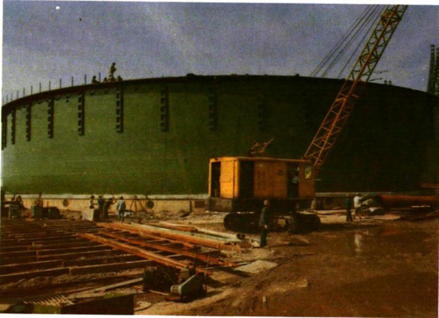
上海宝钢煤气柜
