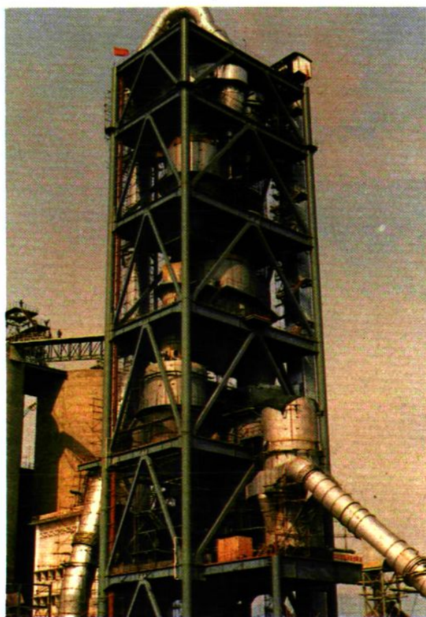
安徽宁国水泥厂予热器
