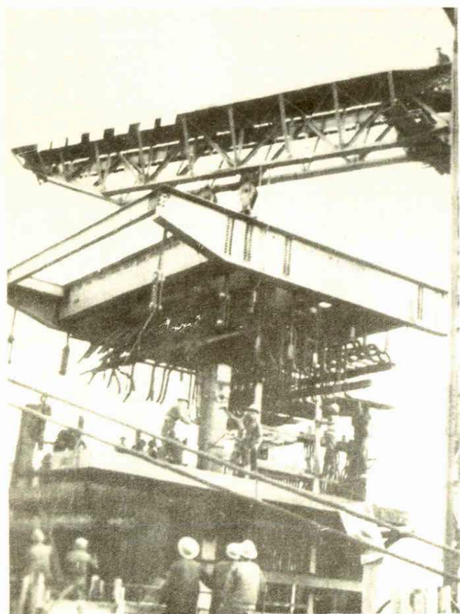
三号炉吊装炉顶
