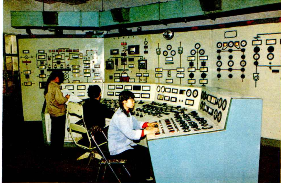
三号机炉操作盘
