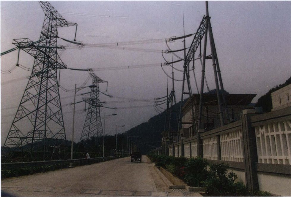
◇ 桐柏抽水蓄能电站 500 千伏出线
