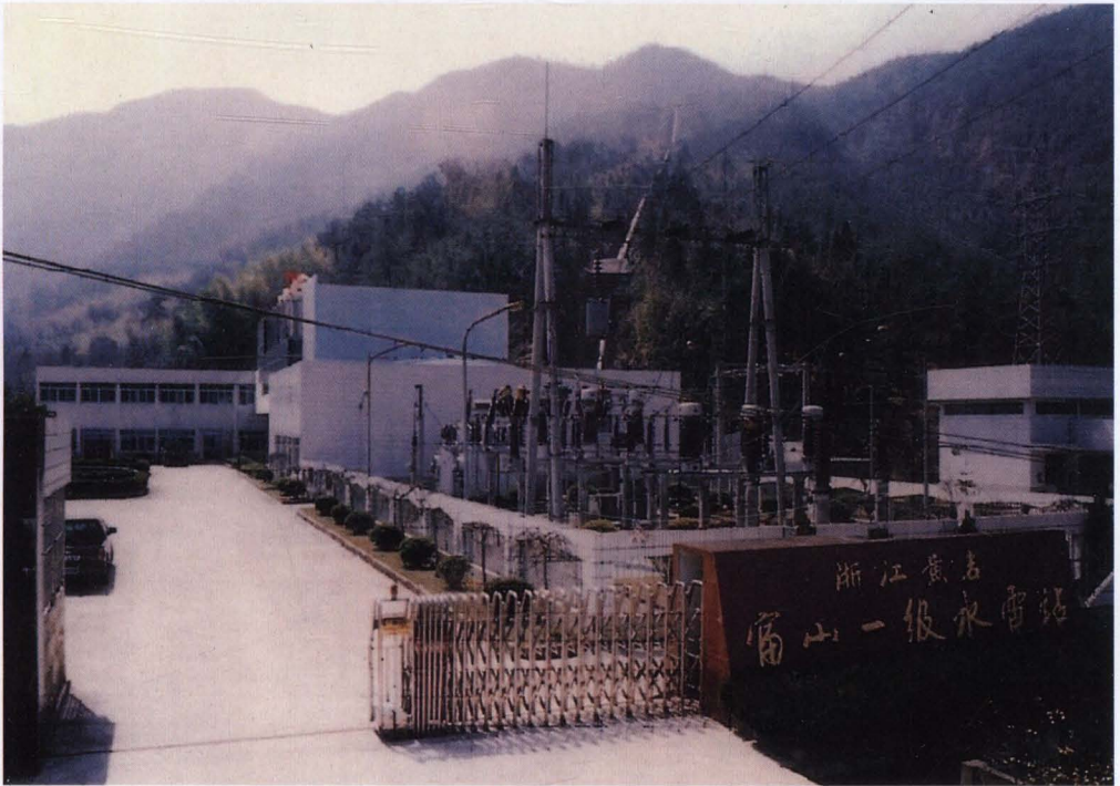
◇富山一级水电站
