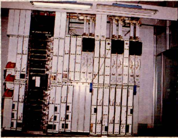
数字微波设备
