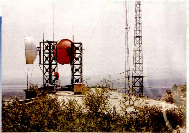
兰州至银川微波干线宁夏段265微波站
