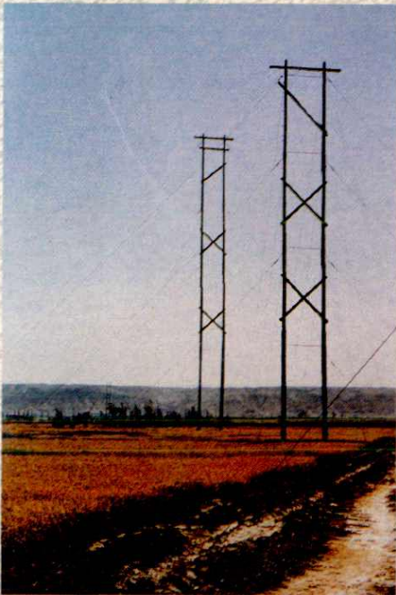
中宁至中卫架空明线 莫家楼黄河飞线
