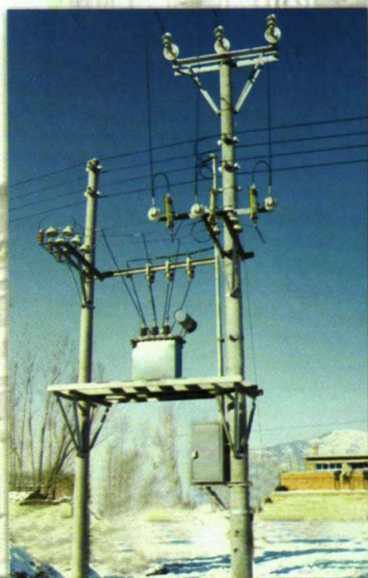
新型标准化配电台区
