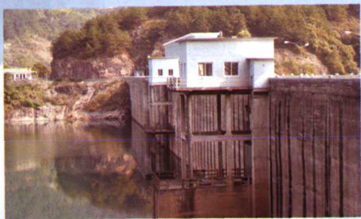
发电输水洞及泄洪底孔进水口
