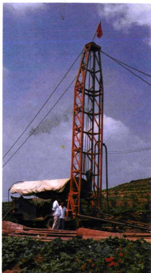
► 沂南县水利局打井队在马头村打深井
