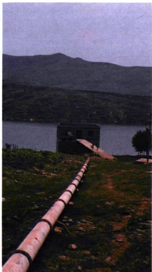
◀ 高湖马眼电灌站
