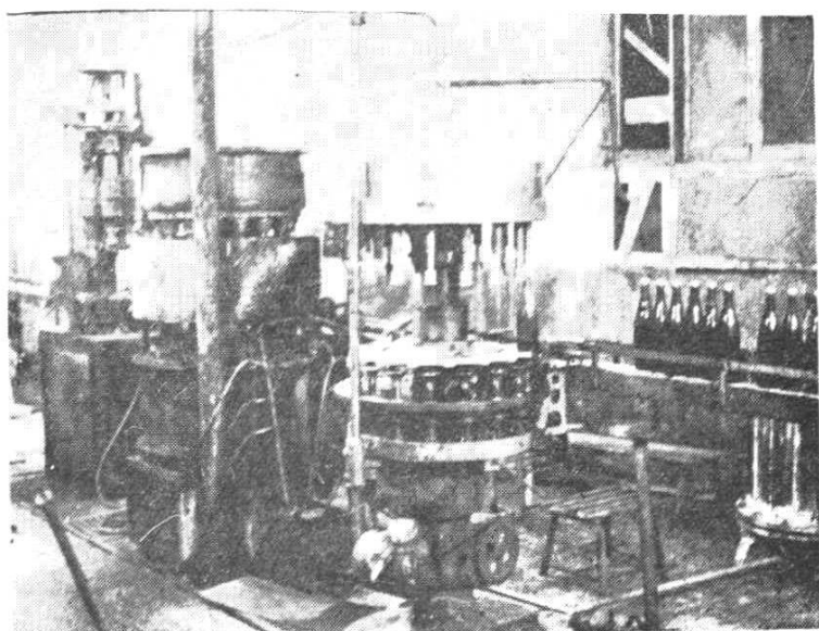
县饮料厂饮料灌装生产线
