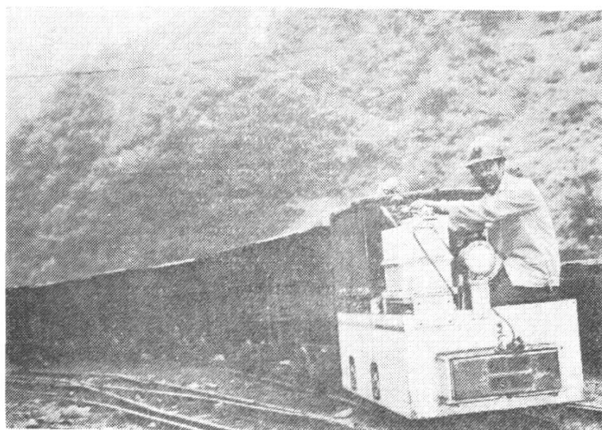
滑石板煤矿电机车运输
