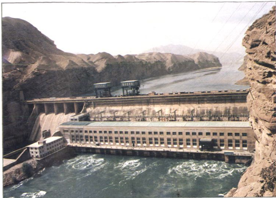
甘肃省建行支持建设的盐锅峡水电站
