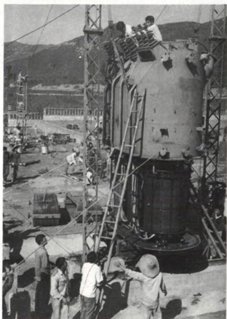
变电队工人在柳州220kV变电站安装主变（1976年）
