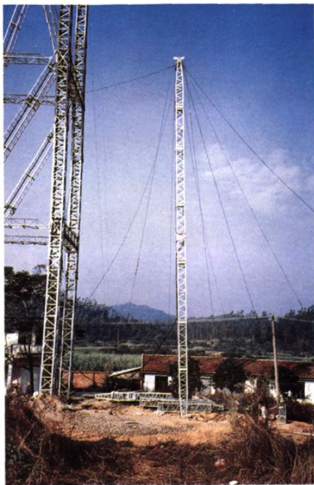
试验测试600mm×600mm×25m铝合金抱杆的性能参数
