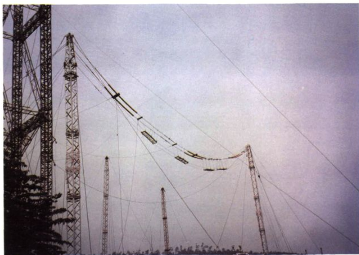
50m完全不停电双柱组合悬索式跨越架
