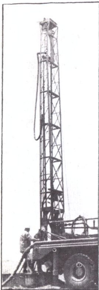
地震队汽水两用钻机正在钻进
