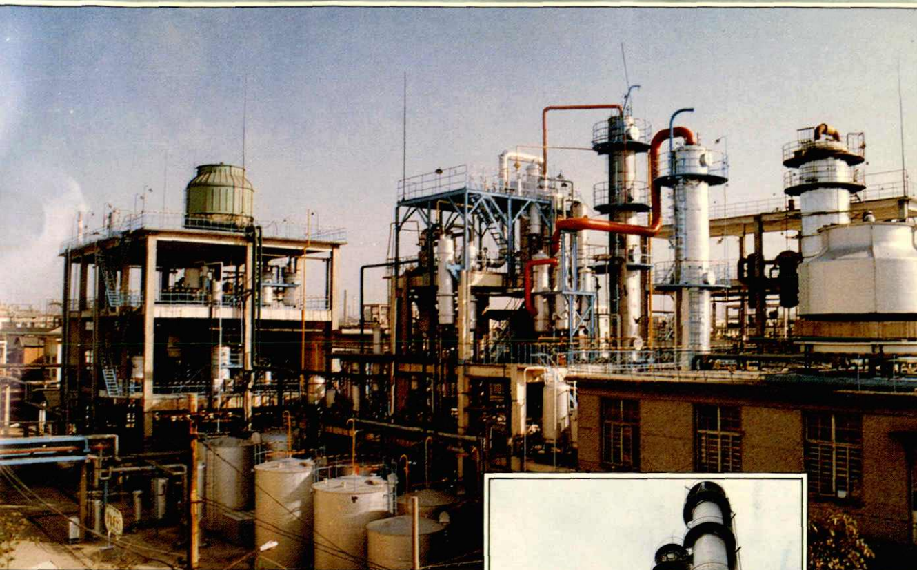
年产 35000 吨硝基苯 加氢还原制苯胺装置
