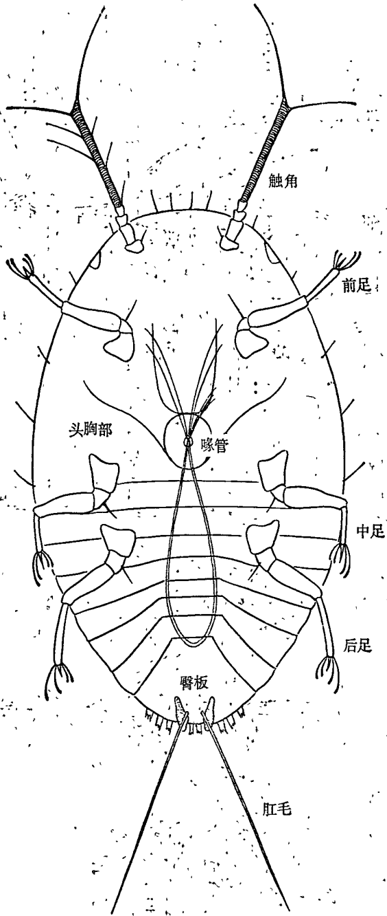
图版 3 介壳虫若虫身体的基本构造
