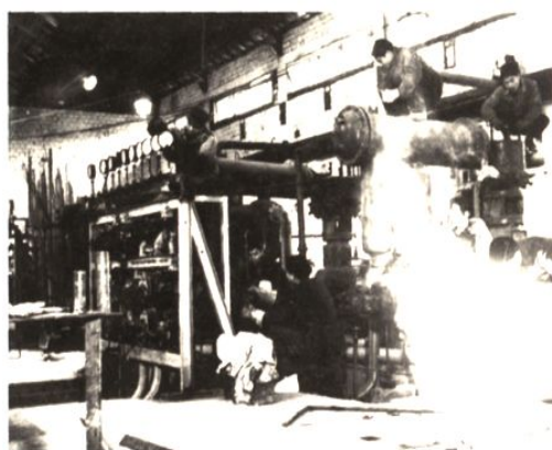
安装高压机
