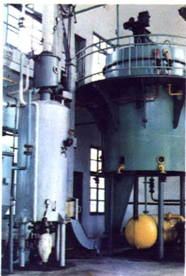
▶ 金华市油脂化工厂 浸出车间
