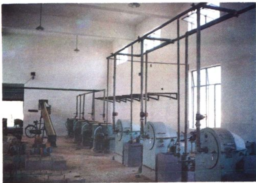
▲ 兰溪市面粉厂变性淀粉车间
