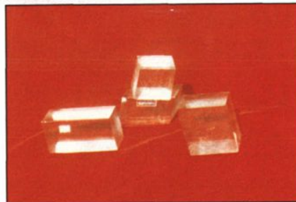
冰洲石
