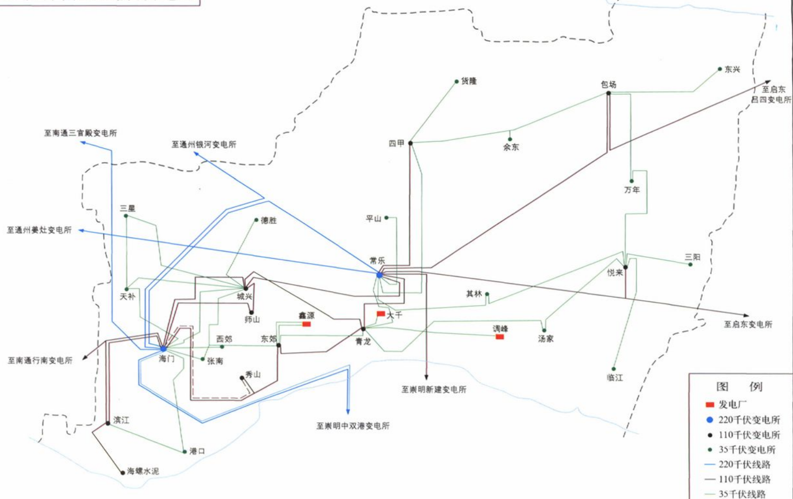
2005年海门市地理接线示意图
