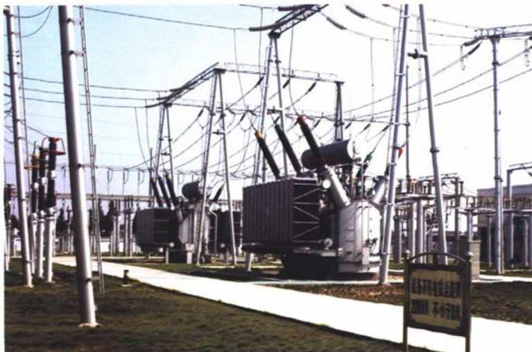
220千伏海门变电所主变压器
