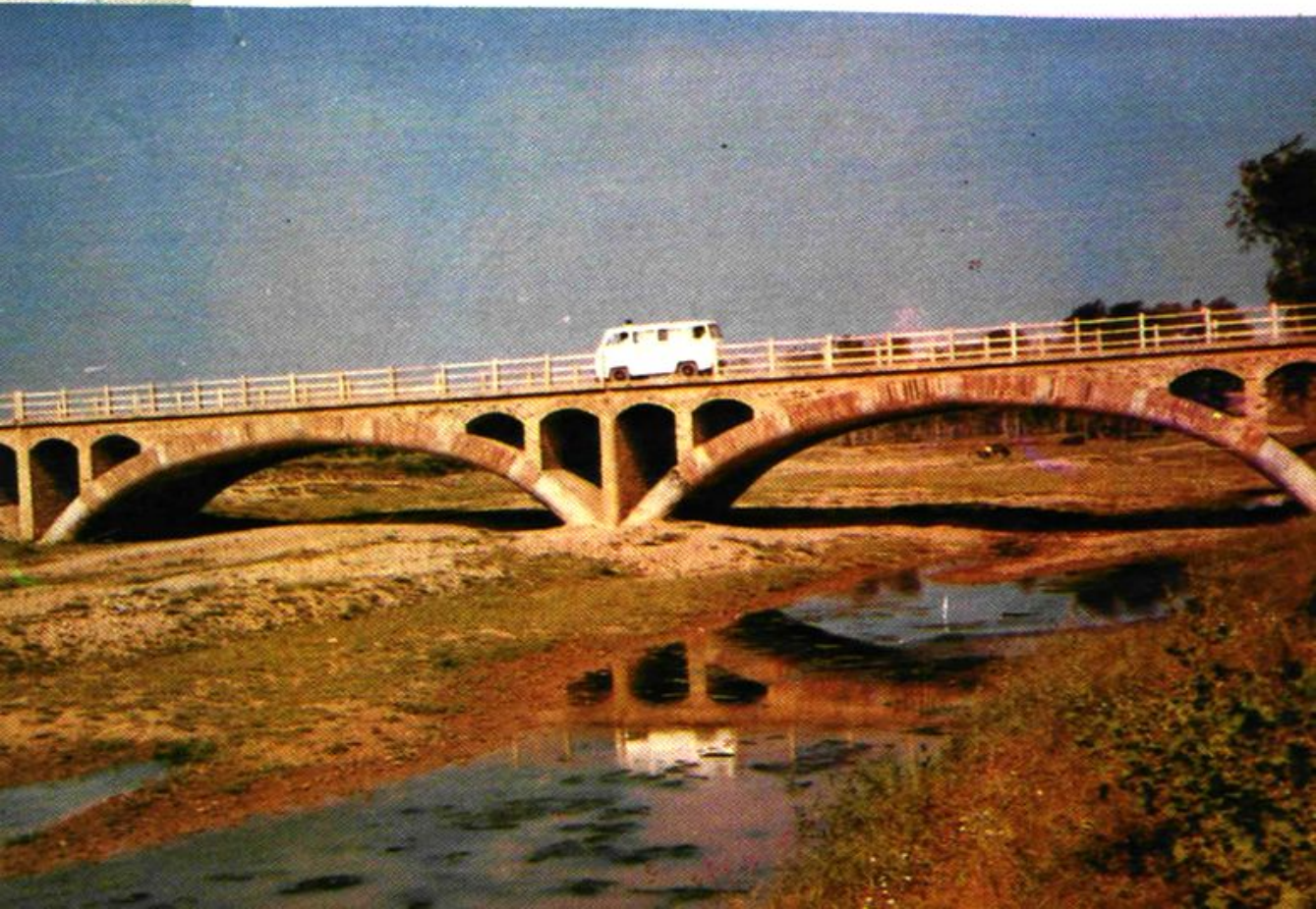
1966年修建的小营子耐火砖筒拱桥
