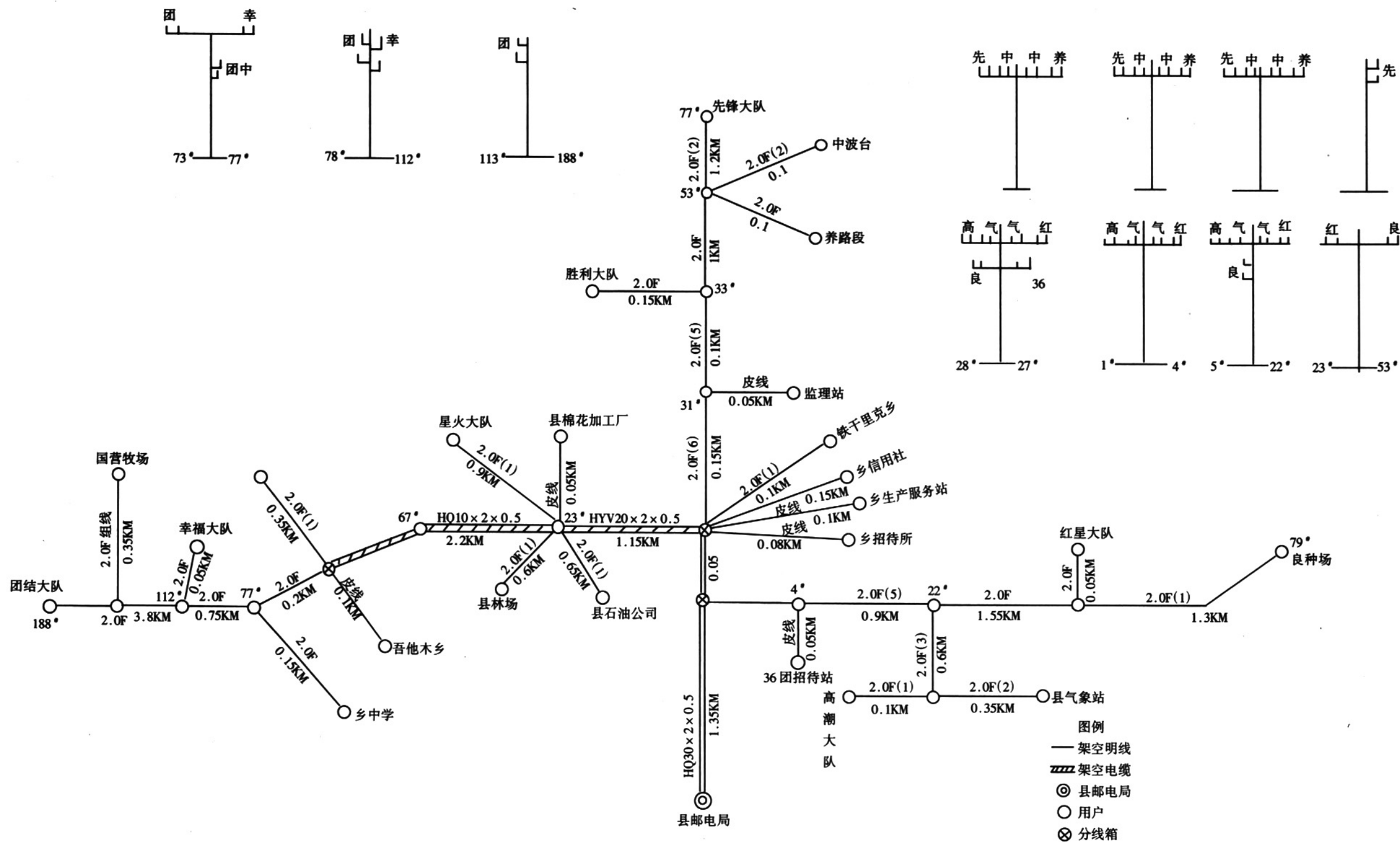
图 3-4 若羌县城效两乡农话线路示意图(1990年7月)
