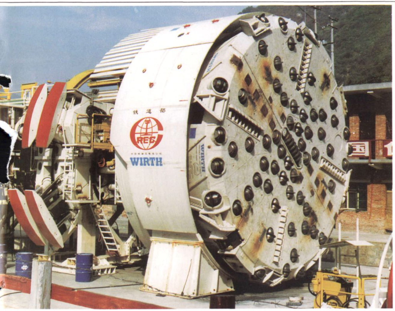
今日掘进机向秦岭开战
