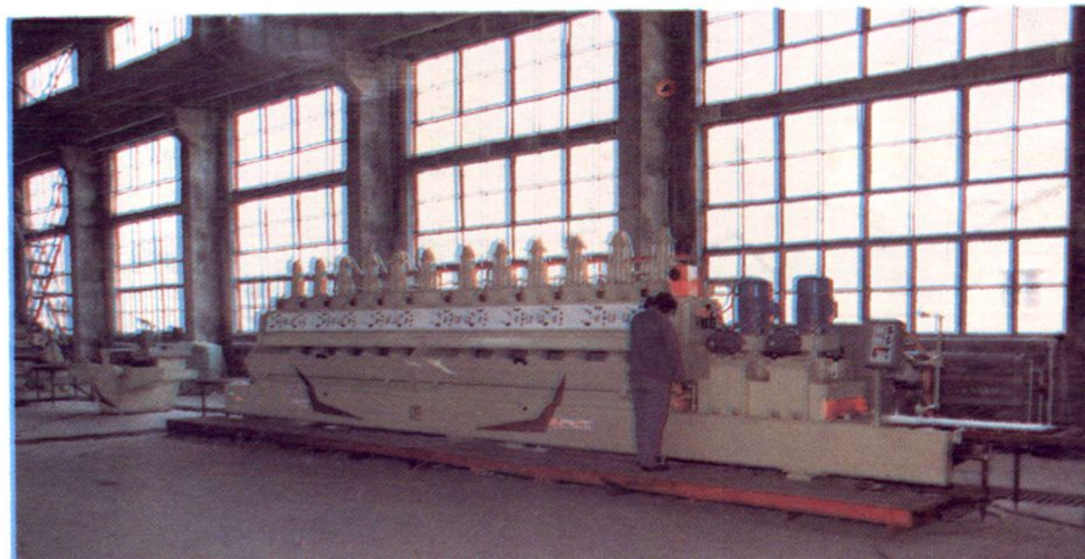
本溪市新型建 材总厂引进意 大利大理石生 产线研磨机
