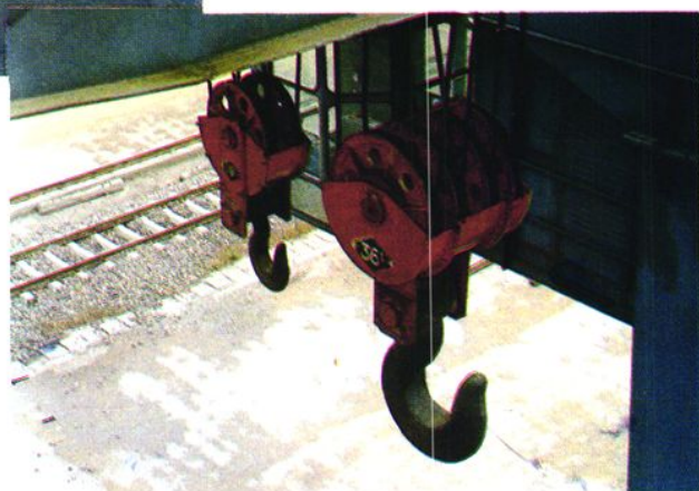
新安装36吨门吊
