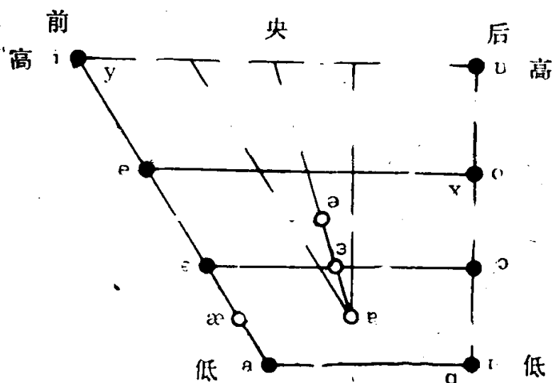
元音图
