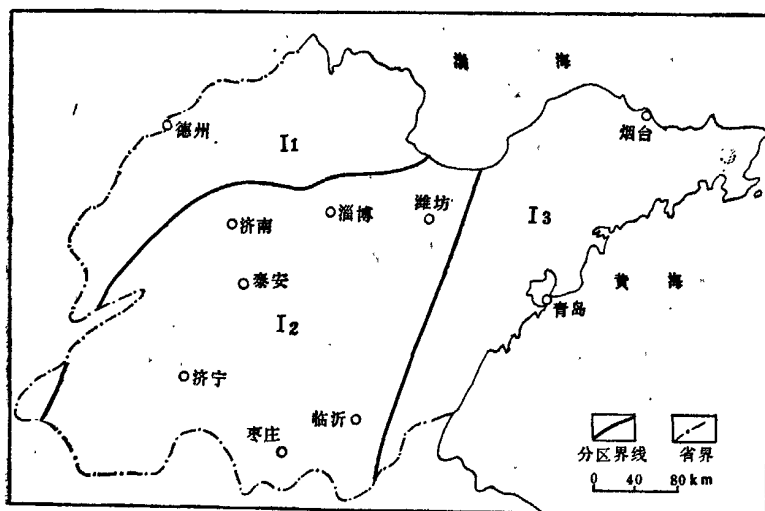
图 I-1-1 山东省地层区划图
