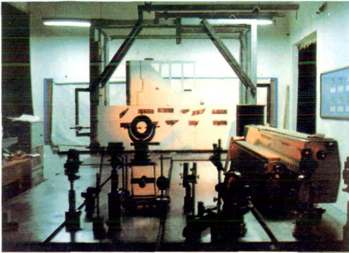
模拟基岩真空产状和模拟地应力技术在结构模型中的应用，为安康电站工程节约400万元投资，该项技术在国内均属首创
