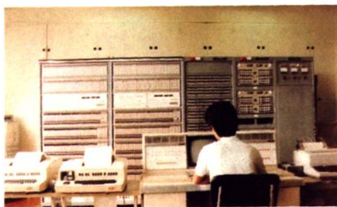
1985-1989年使用的布控140线（后扩容为280线）用户电报及低速数据交换机。
