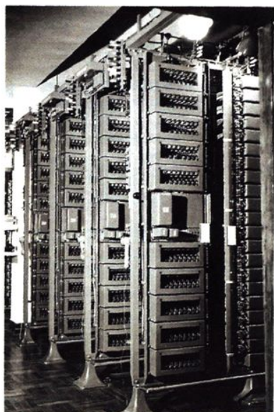
1963年6月9日 在东街口邮电 大楼二楼开通 了国产ATC- 47式步进制 市话自动交换机。 电话号码从4 位升为5位。
