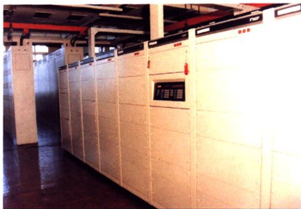
1982年11月27日福州在全国率先开通万门程控。图为设在东街口邮电大楼二楼的东街母局（8000门）机房。
