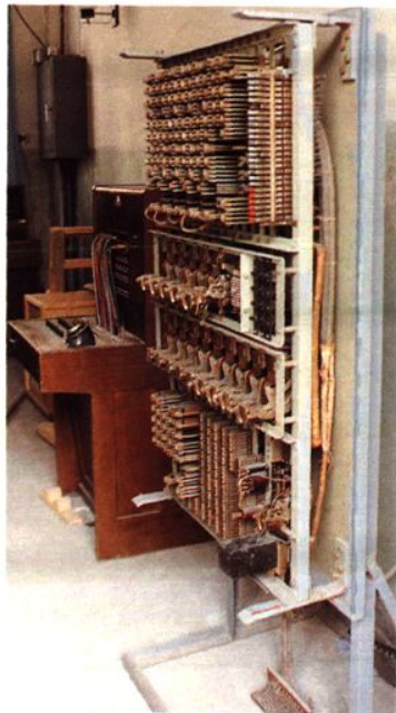
早期共电市话交换机。
