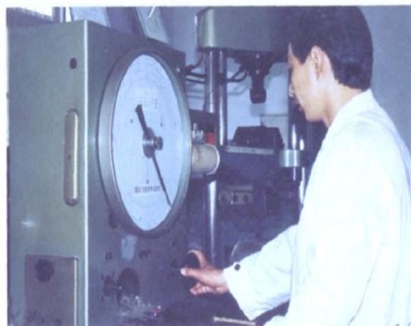
▼ 拉力弯曲试验
