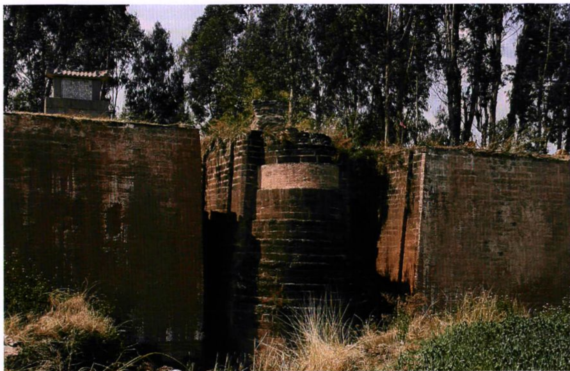
姚安大石坝元代水利工程
