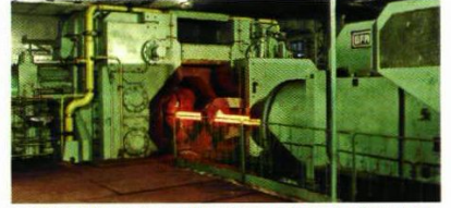
抚钢股份公司锻造厂1000吨精锻机
