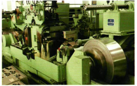
大连精密合金有限公司高精度20辊冷轧机
