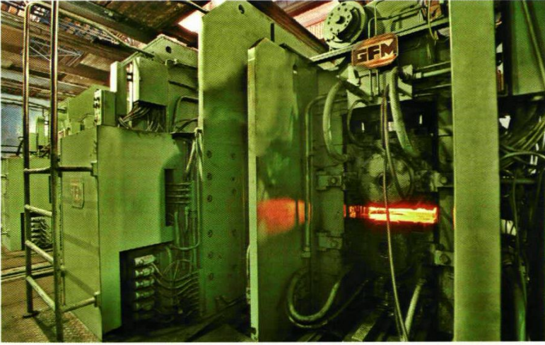
抚钢股份公司精轧厂WF-5-40型方扁钢精轧生产线
