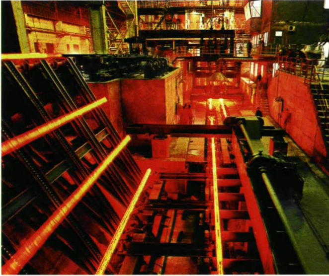
大连金牛股份公司第一炼钢厂连铸机
