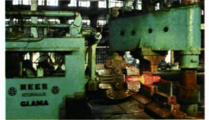
抚钢股份公司锻造厂2000吨快锻机
