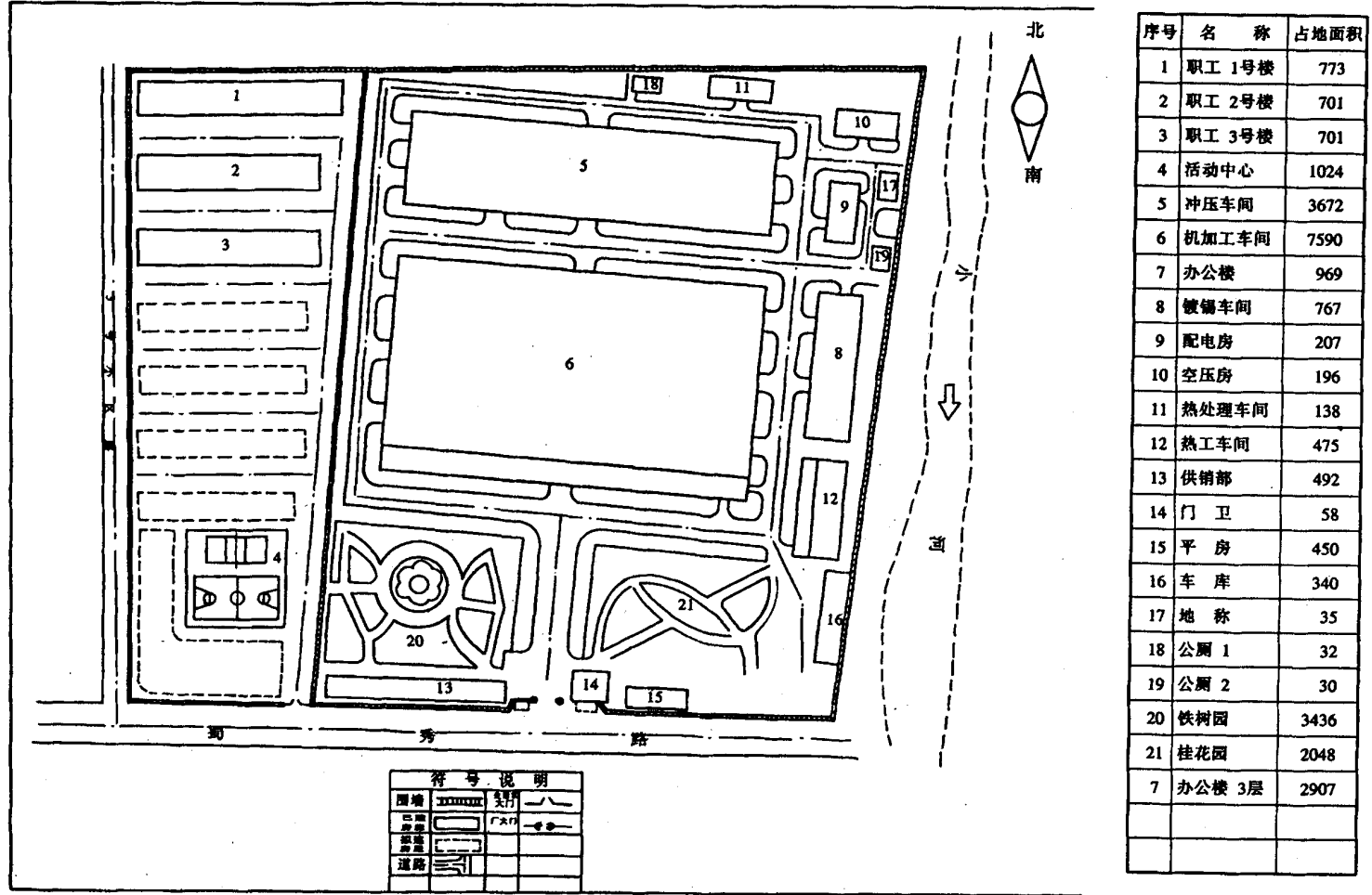
四川飞虹轴瓦股份有限公司(开发区)总平面图 (1996年)
