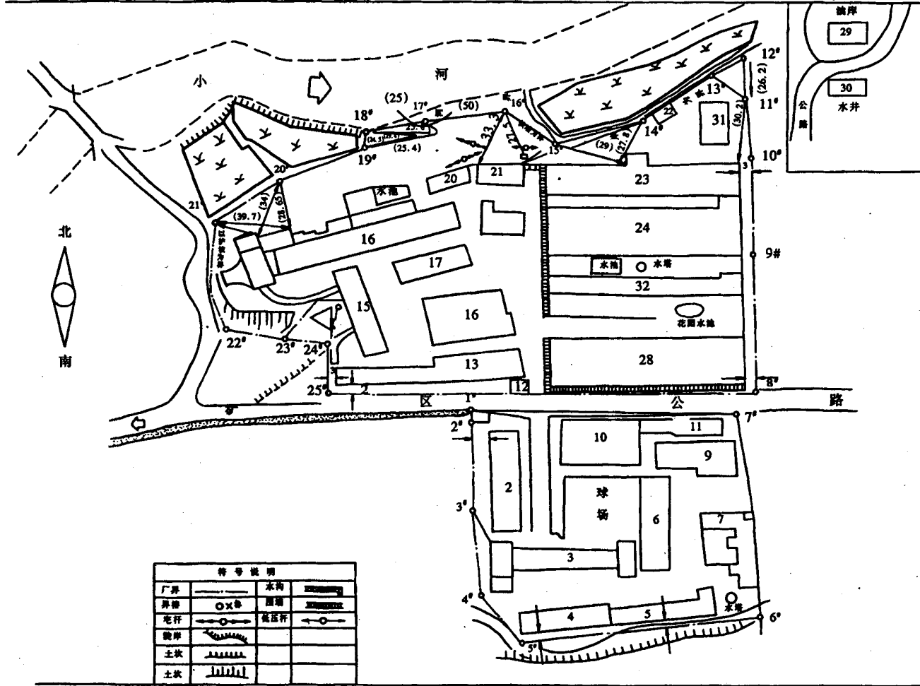
四川省遵义市轴瓦厂厂区(新厂)总平面图(1990年)
