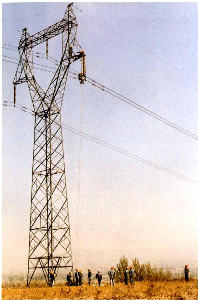
带电检修 220 千伏线路
