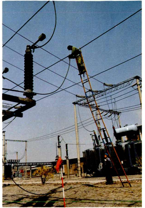
110 千伏带电拆接引线
