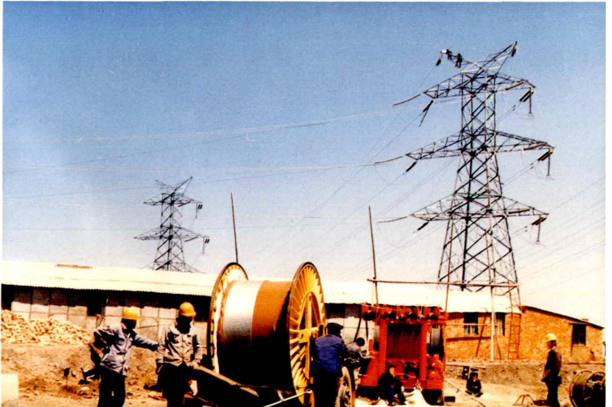
架设 220 千伏线路
