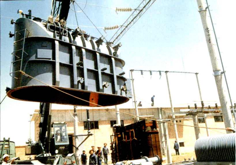
安装 110 千伏黄寨变电站主变压器
