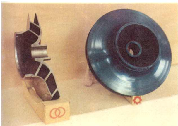
高压锅炉给水泵泵轮
