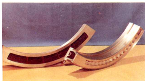
汽轮机高压喷嘴
