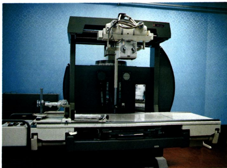
多轨迹断层床HL - 31 主要用途：各种断层及拍片
