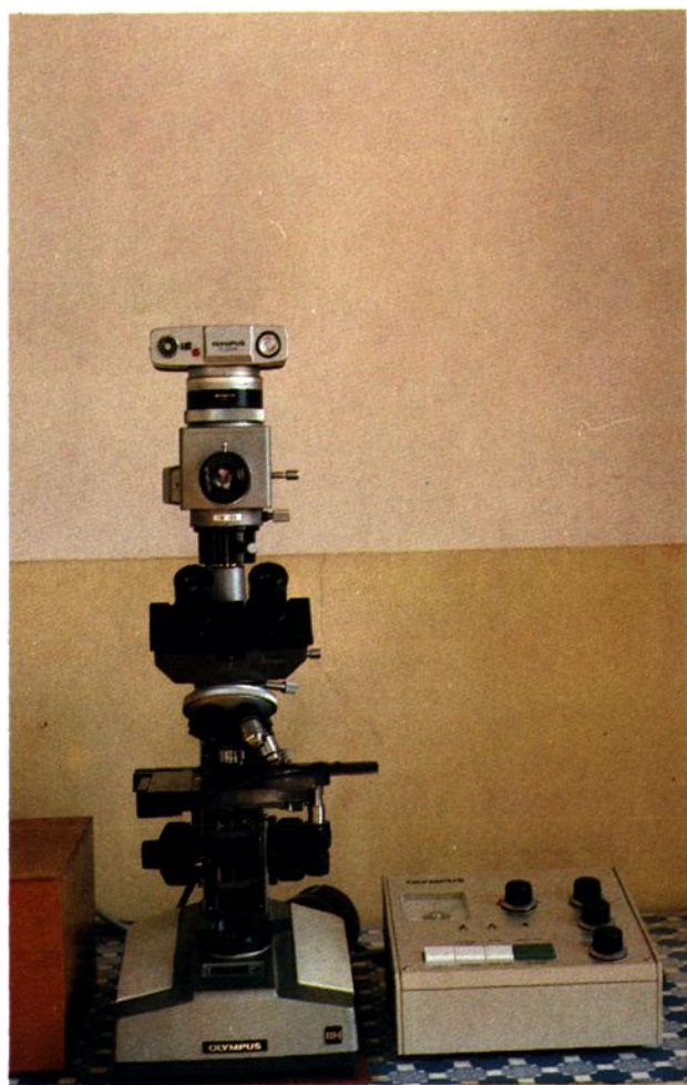
显微镜照相机BH-PM-10A 主要用途：黑白、彩色显微镜照相
