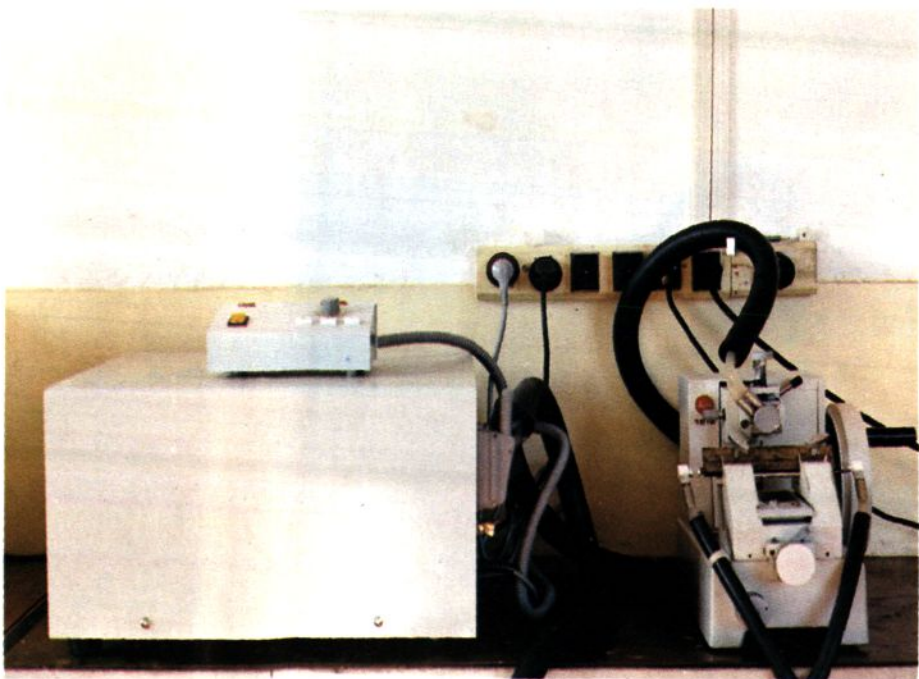
组织切片机Leitz1512连接Kryom at 1700冷冻装置
