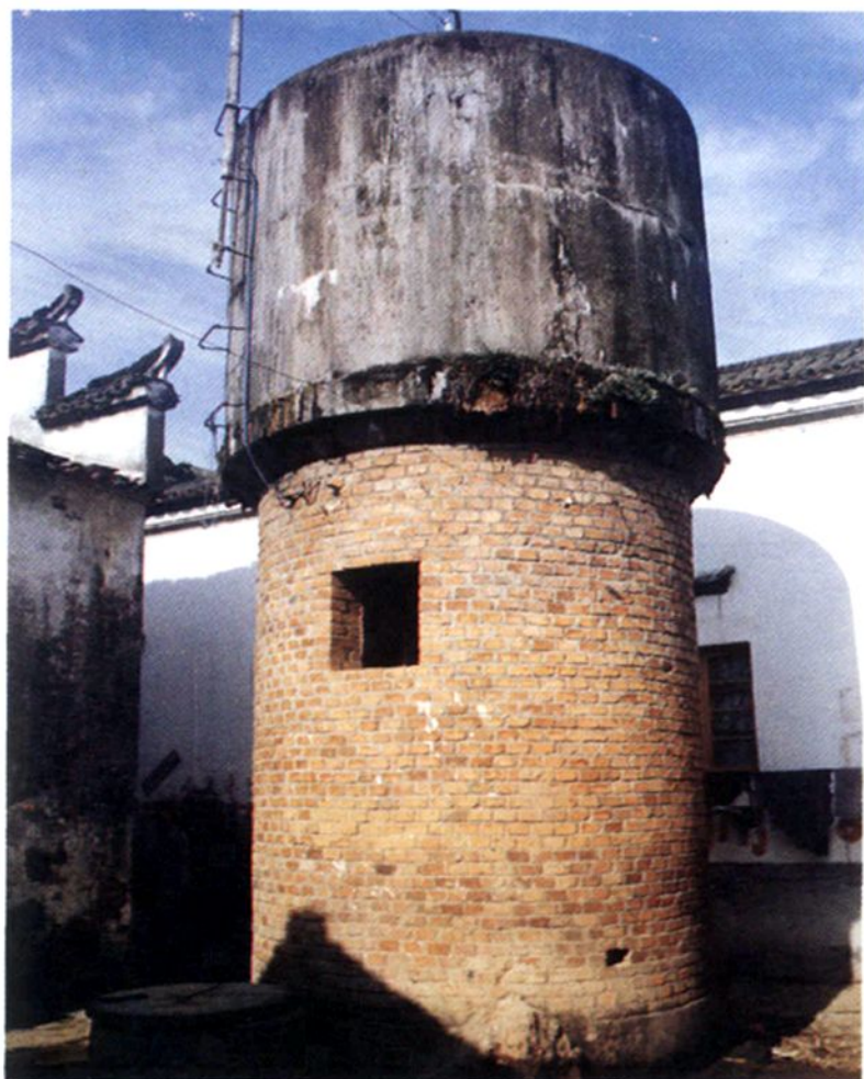
1979年采用聚乙烯塑料管建造的金华县第一座水龙头到户农村自来水厂，在洋埠镇上陈村建成。
