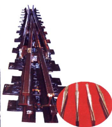
蓝星机械制造的铁路辙叉芯轨
