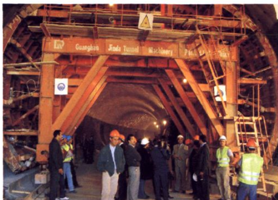
广汉金达隧道机械为摩洛哥王国设计制作的 双线铁路隧道台车
