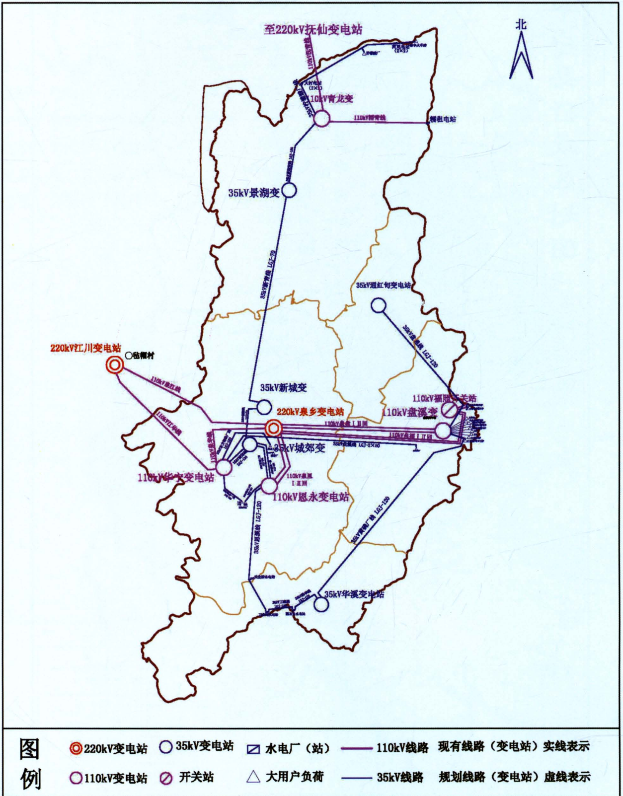
2014年华宁县电网地理接线示意图
