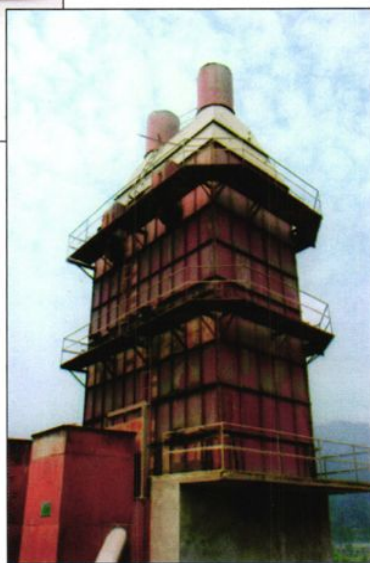
▲ 3×11M机窑电收尘器
