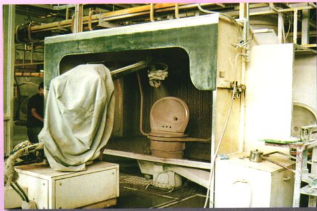
▲ 机械手喷釉(1995年)
