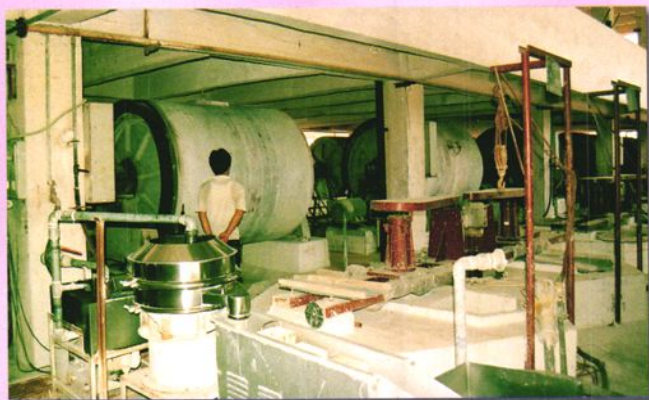
▲ 1998年球磨机加工原料
