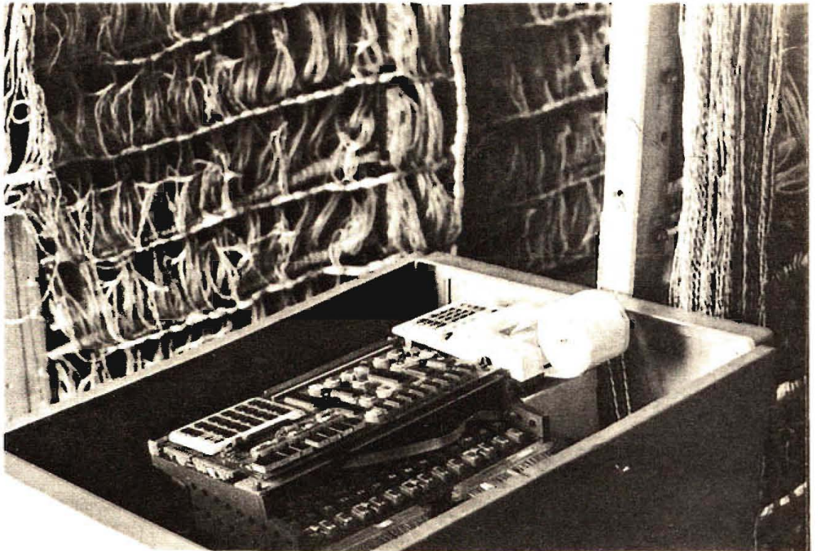
我国第一台铁路“驼峰”信号电路 微机监测装置 薛贵宝 摄
